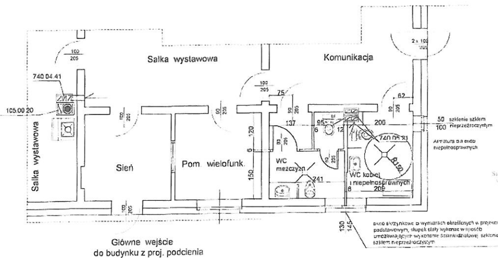
RZUT PRZYZIEMIA 1:50
